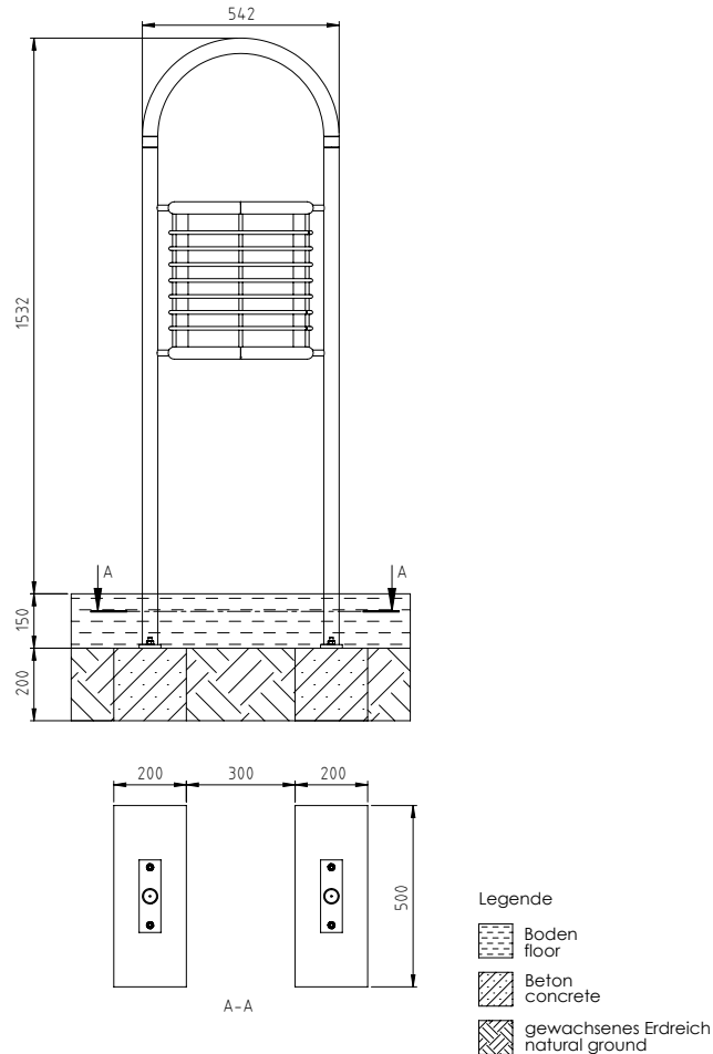
Skizze 2: Fundamentplan
